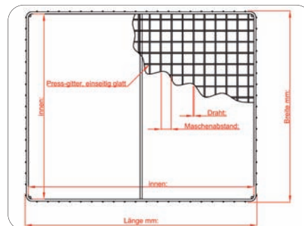
Drahtgitterkorbboden Typ RPK1
