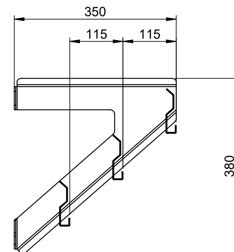
SCHNITT A-A
