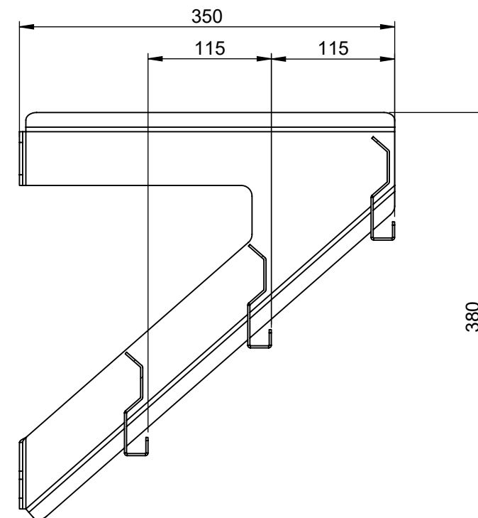
SCHNITT A-A SKALA 1 : 5
