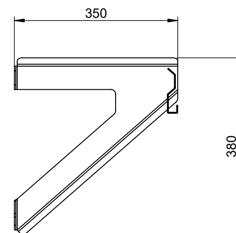
SCHNITT A-A
