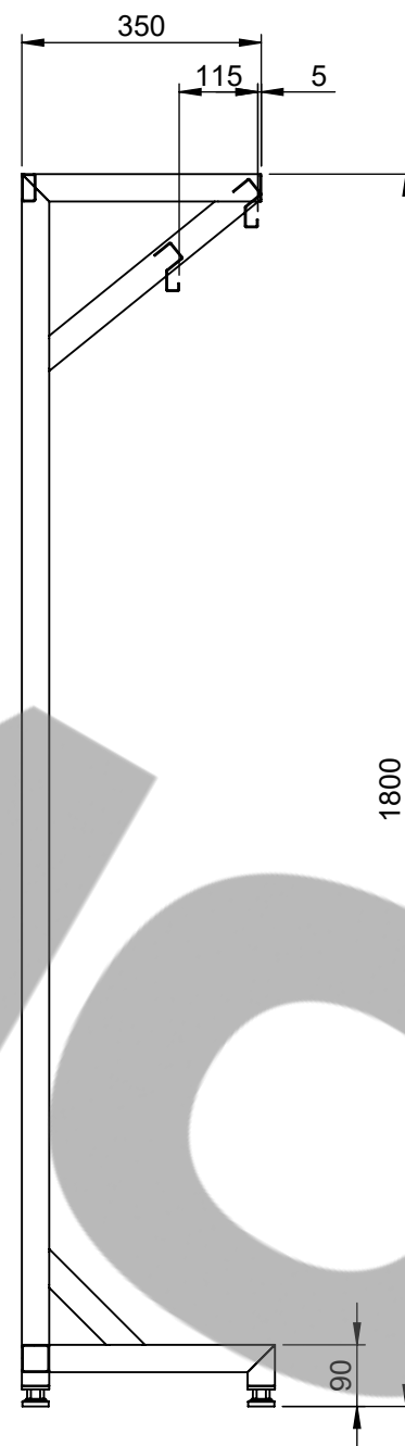
SCHNITT A-A
