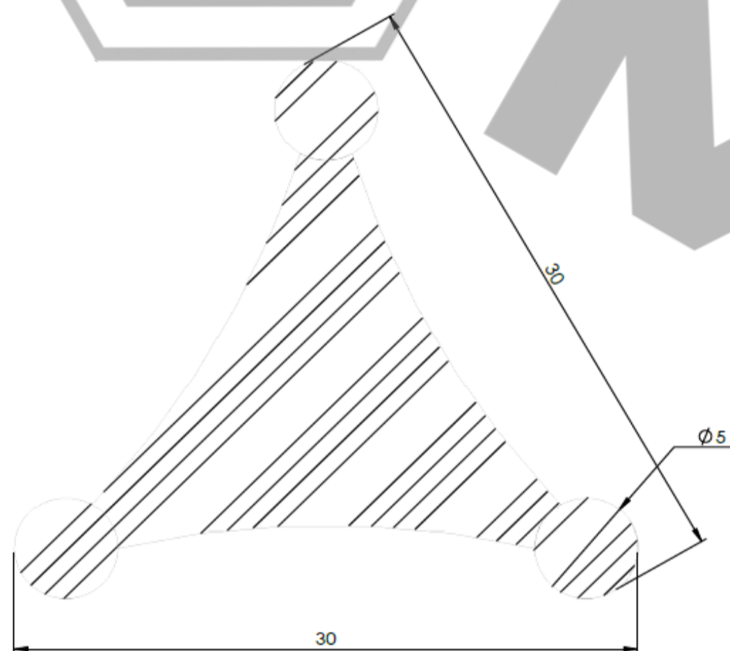
SCHNITT A-A
