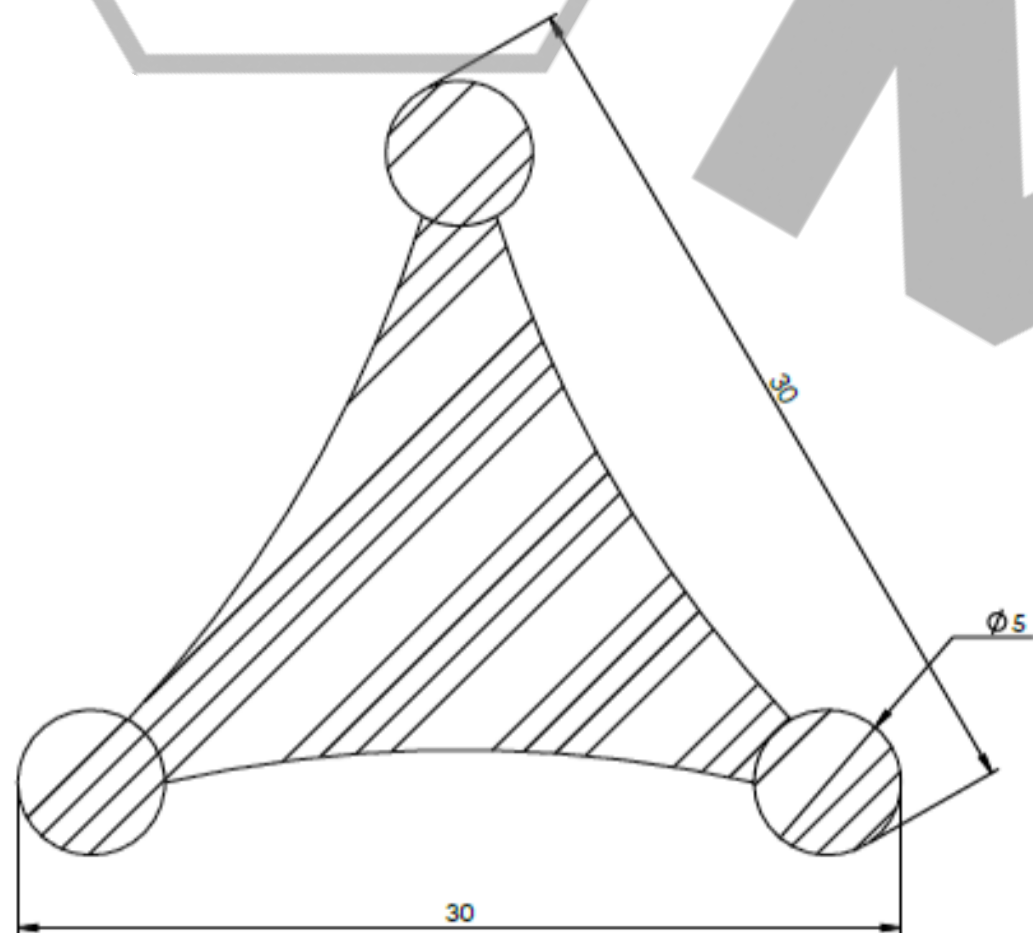
SCHNITT A-A
