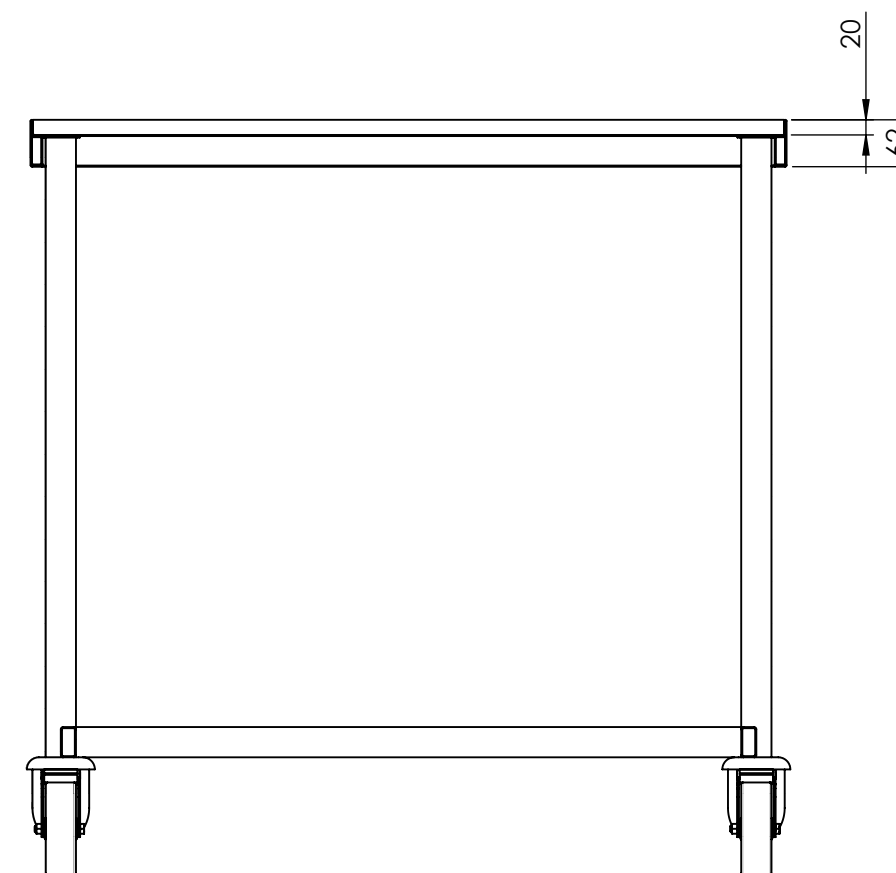
SCHNITT K-K
