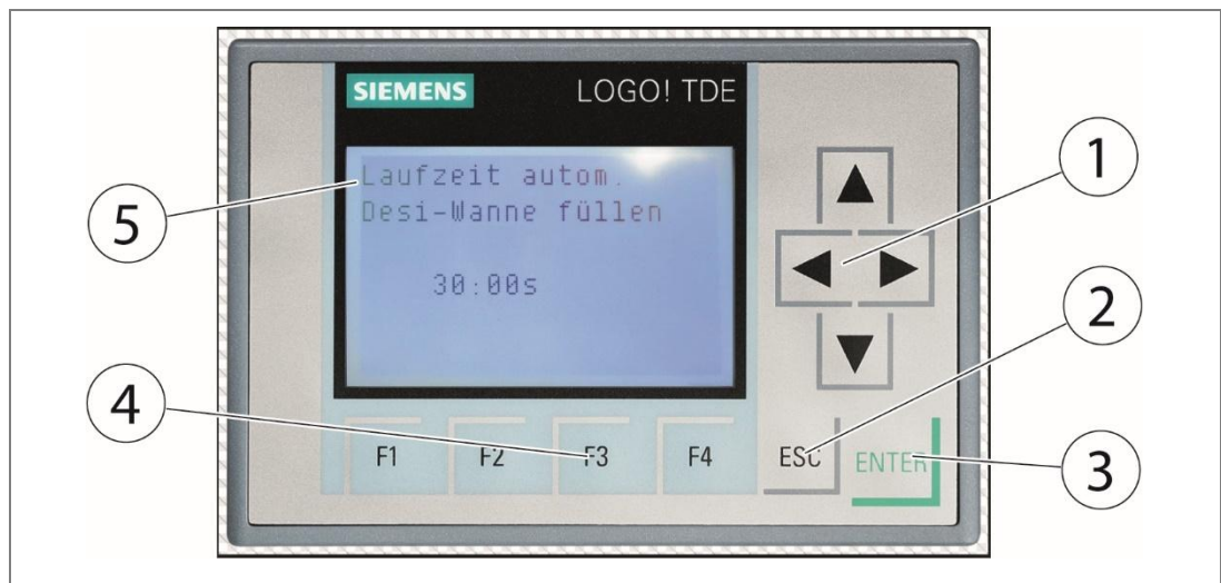
Abb. 8: – Siemens LOGO! F3
