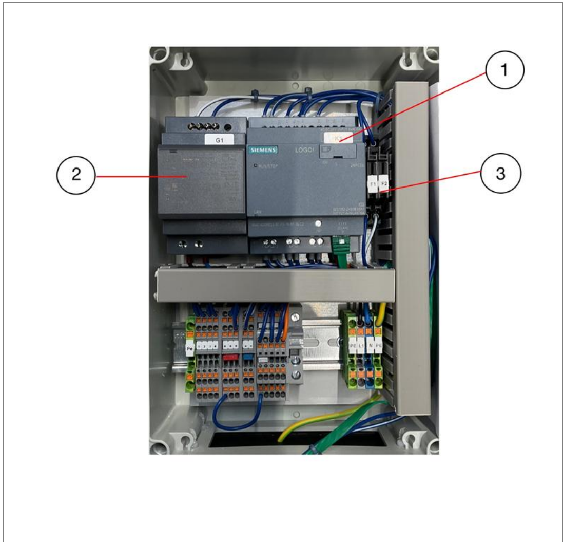
Abb. 12: – Steuerungskasten
